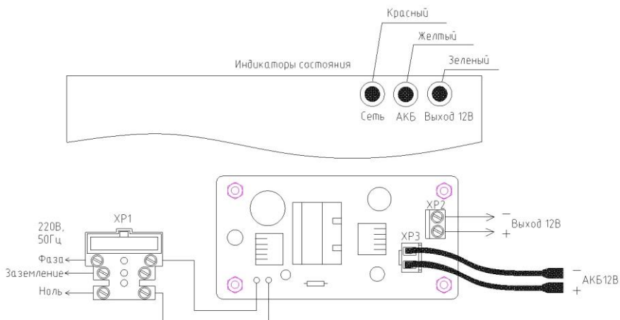
Рисунок 1 Схема подключения Optimus 1230-RM-7
